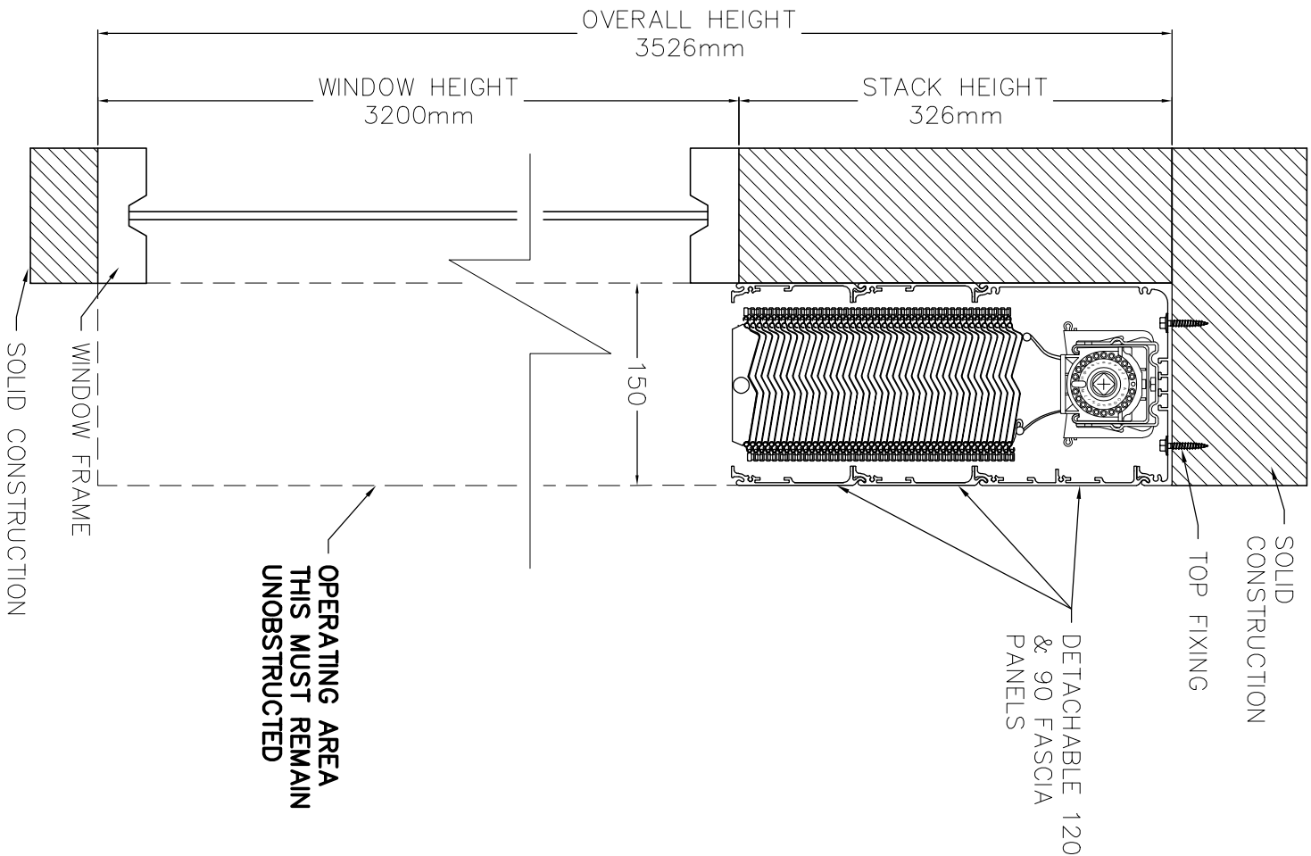
TOP FIX
